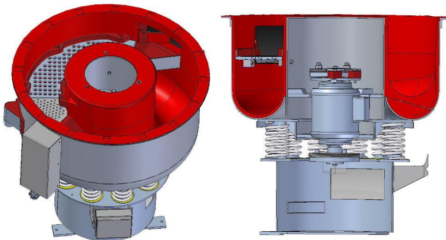
Hochleistungs-Rundtrogl Gleitschleifanlage VA
